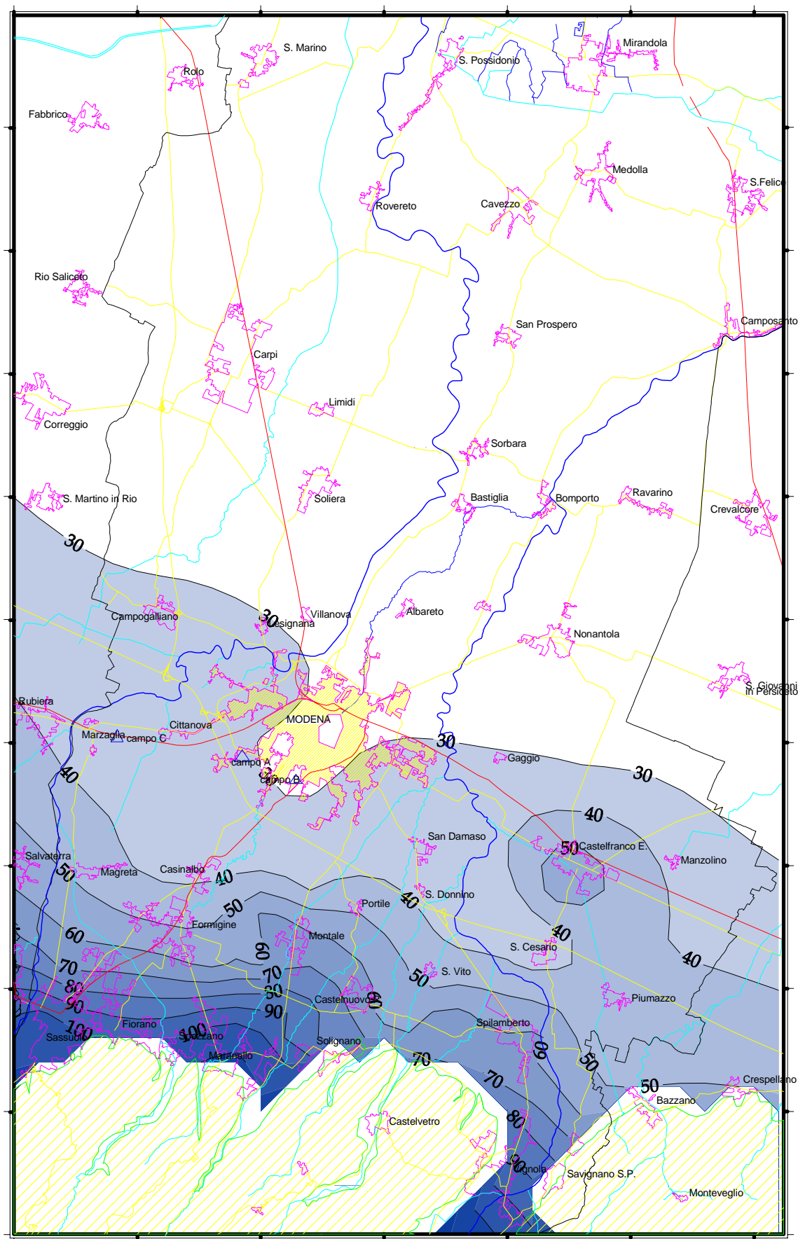
Figura 12 - Piezometria (m. s.l.m.) media anno 2004.
