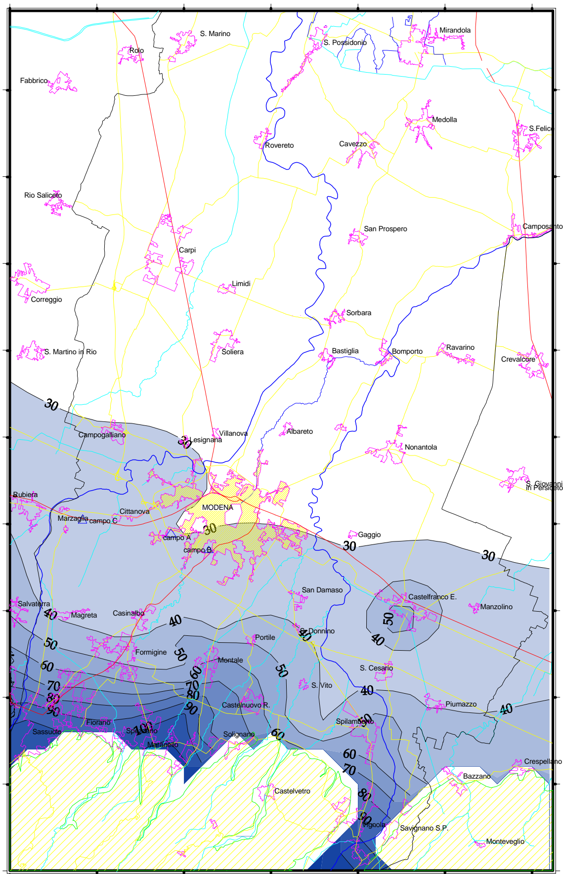
Figura 11 - Piezometria (m. s.l.m.) media anno 2003.
