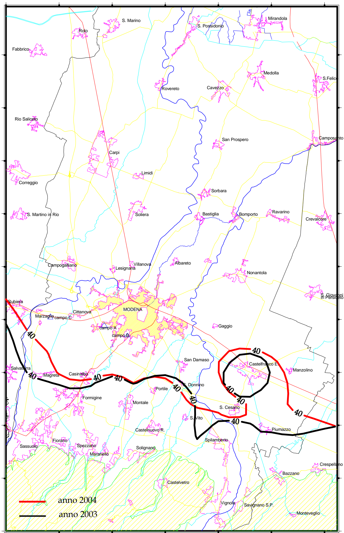
Figura 14 - Piezometria (m. s.l.m.) confronto medie anni 2003 e 2004 - isopieze dei 40 m.
