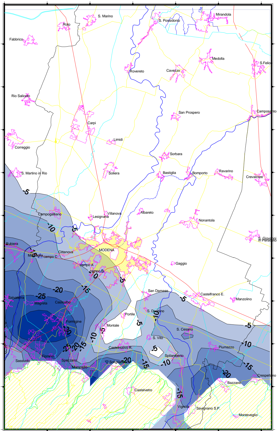
Figura 15 – Soggiacenza (m) media anno 2004.
