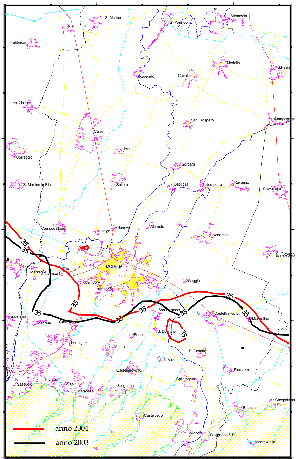
Figura 13 - Piezometria (m. s.l.m.) confronto medie anni 2003 e 2004 - isopiezies dei 35 m.
