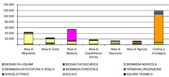
Potenziale energetico (Tep/anno)
